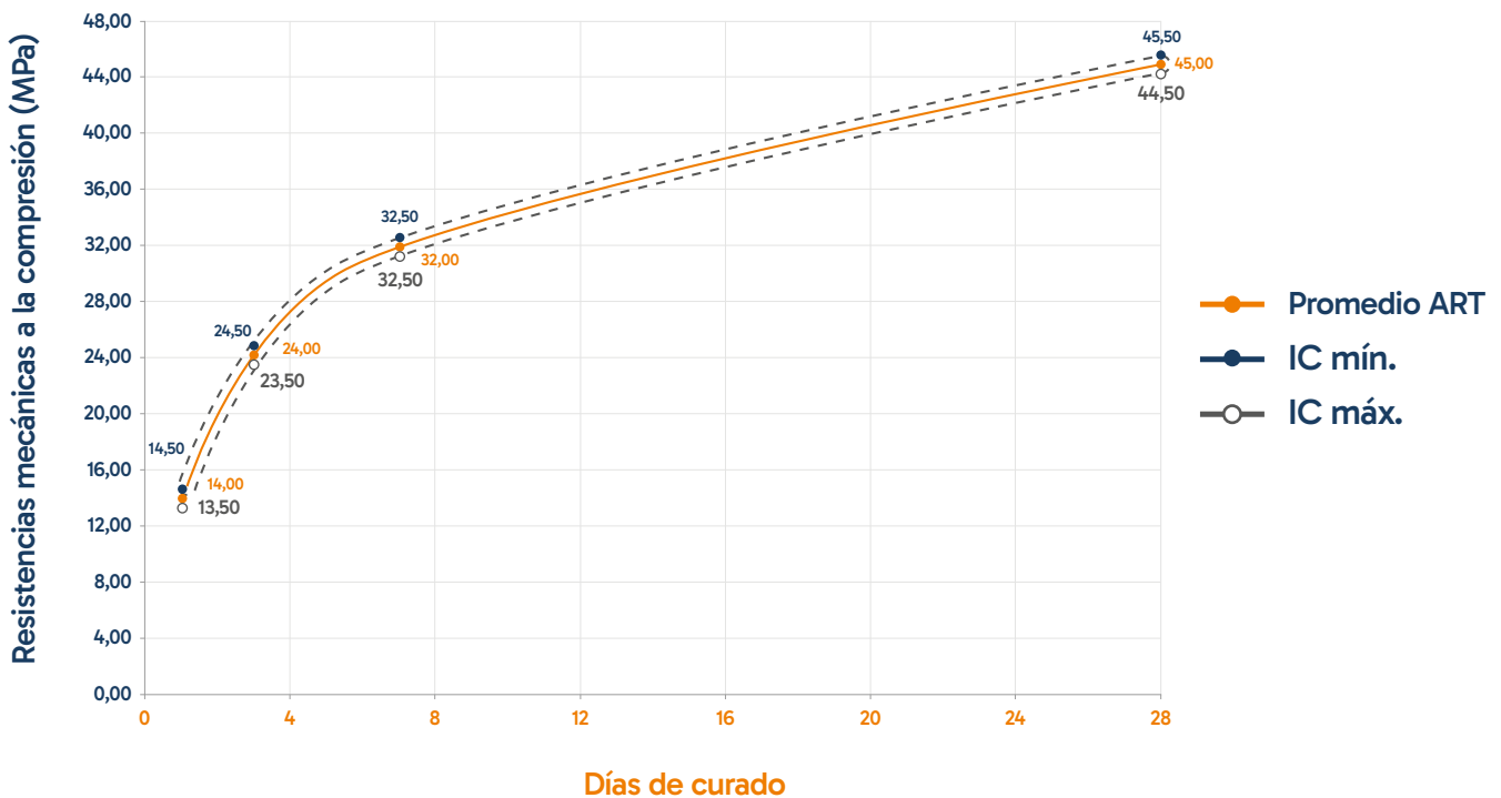
Curva de desarrollo de resistencia Cemento Estructural Tipo ART San Marcos
